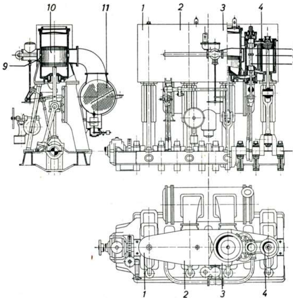
Fredriksstad Mek. Verksted dampmotor.
