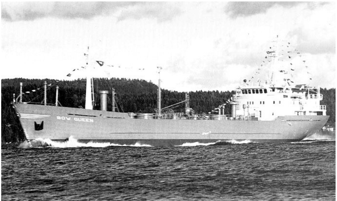
BRG51619690220001 BOW QUEEN. Foto fra boka Båter bygd og levert av Trosvik Verksted.
