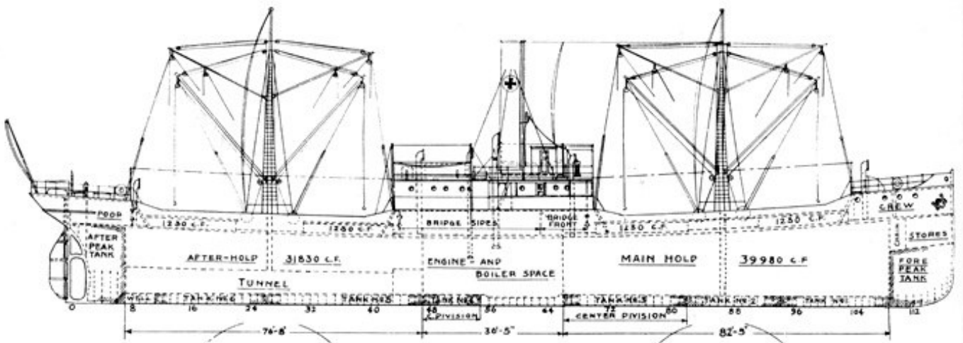
TBG13119140120001 PORTIA. Tegning fra boka -her byggedes skibe av Finn R. Hansen.
